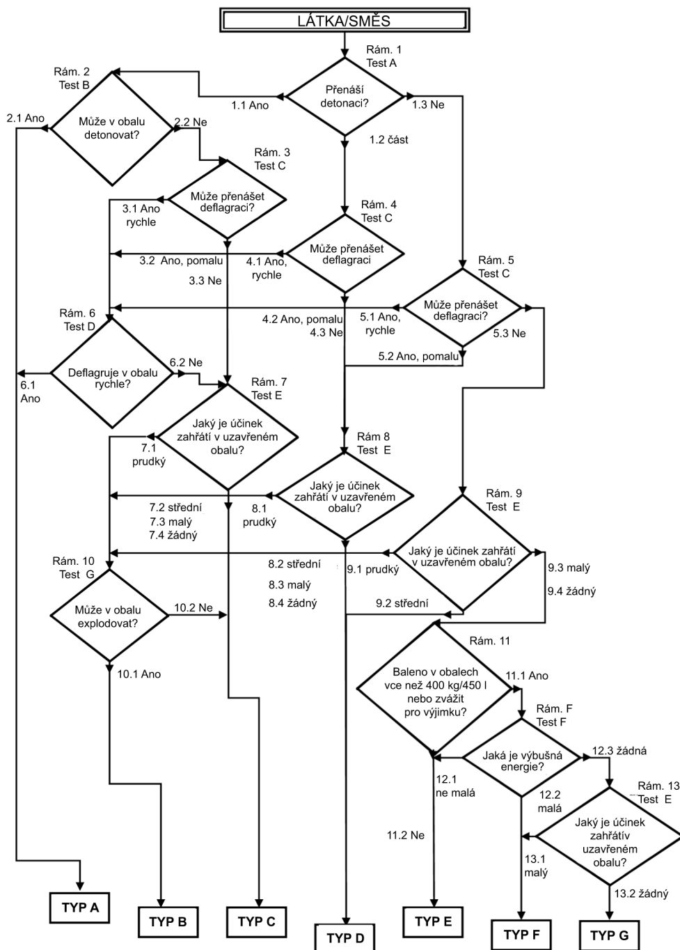
Obrázek 2.15.1 Organické peroxidy
